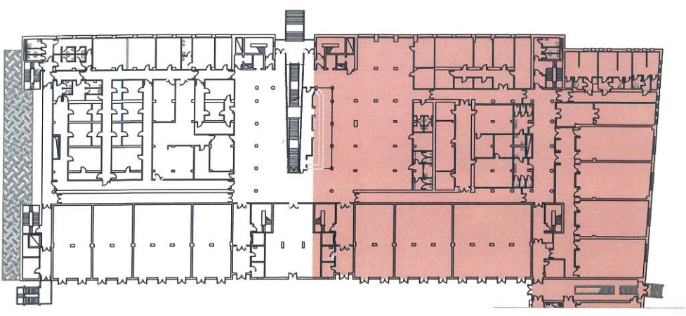
EDIFICIO FARMACIA Planimetria Secondo Livello_Basamento
