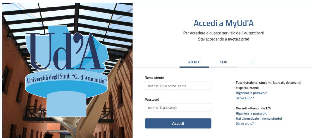
Figura 1: Autenticazione
