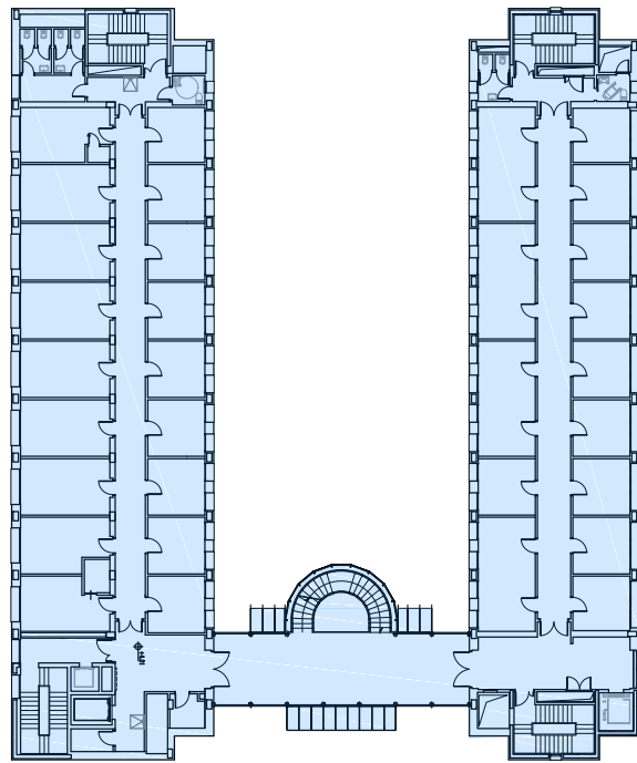
EDIFICIO FARMACIA Planimetria Secondo Livello Elevazione
