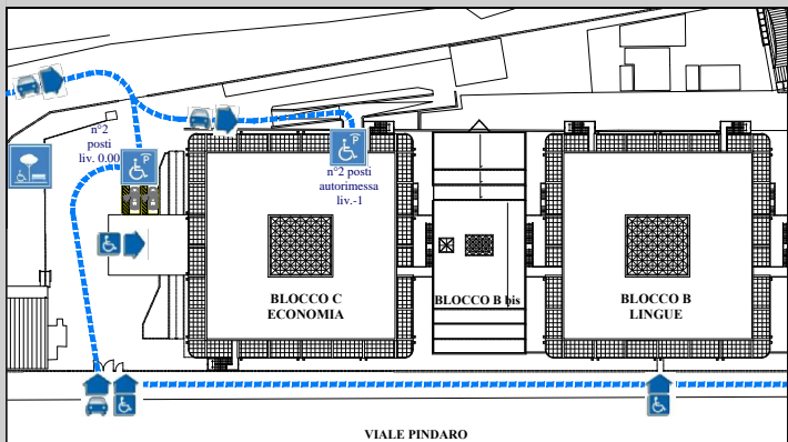
Ingresso carrabile_parcheggio_accessibilità
