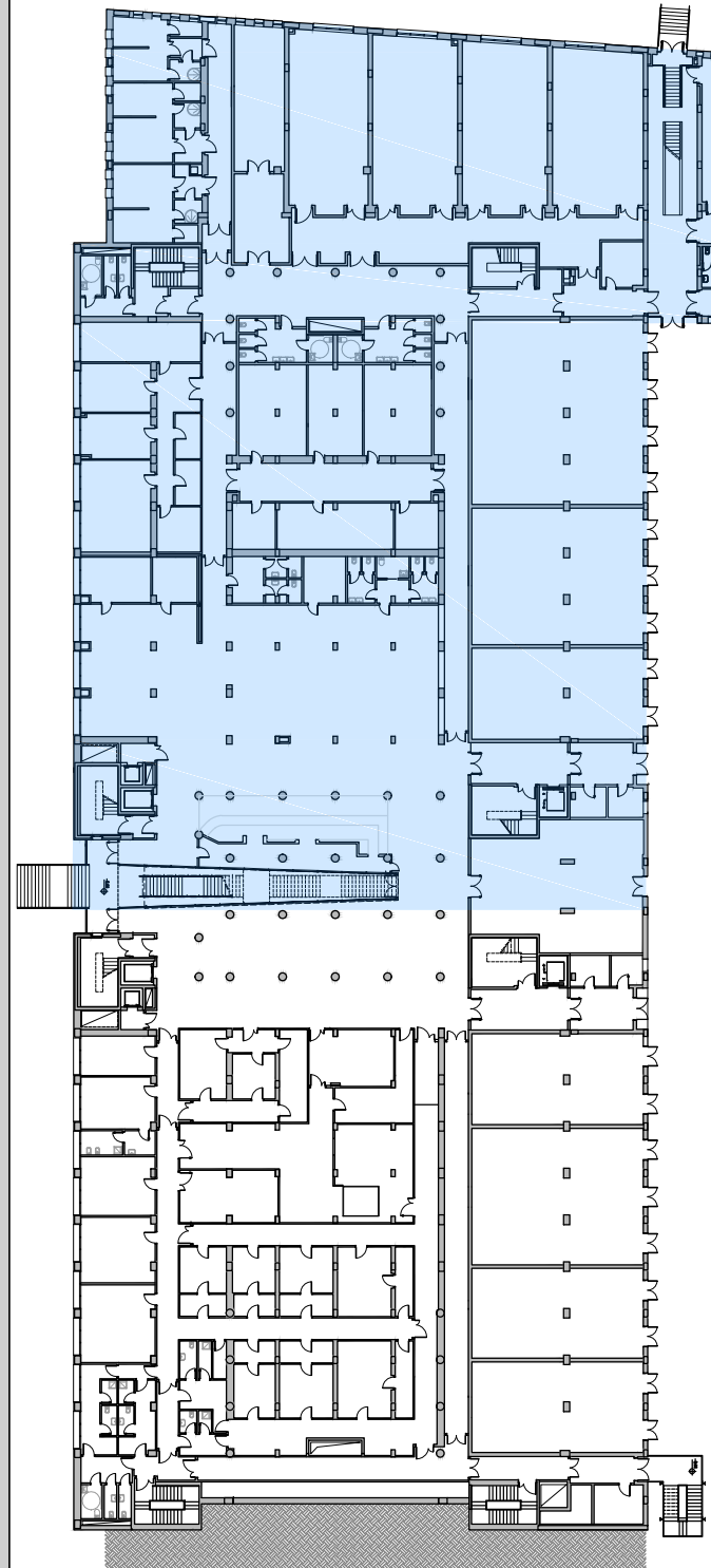
EDIFICIO FARMACIA Planimetria Secondo Livello_Basamento
